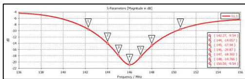
Gambar 9. Grafik S-Parameter Simulasi
