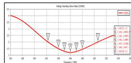
Gambar 10. Grafik VSWR Simulasi
