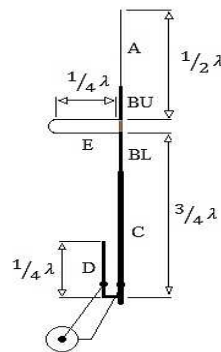
Gambar 5. Konstruksi Antena Super J-Pole
