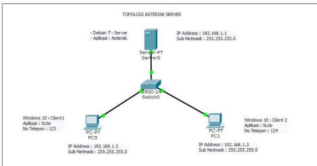
Gambar 4. Konfigurasi Asterisk
