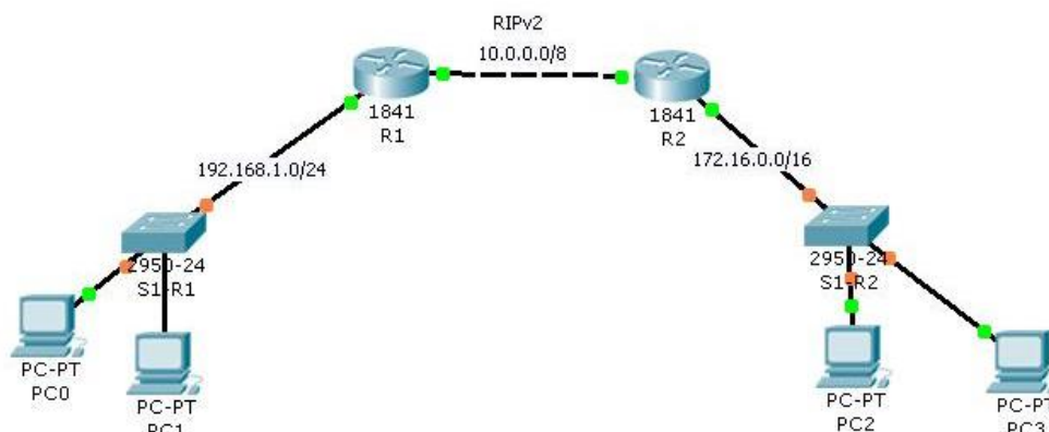
Gambar 3. Konfigurasi RIPv2
